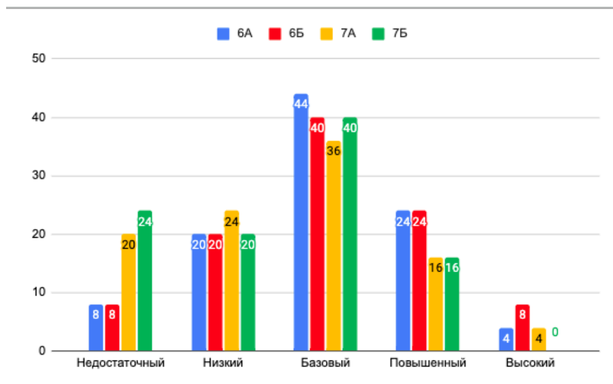
Диаграмма. Результаты внутренней диагностики математической грамотности в 6–7-х классах
